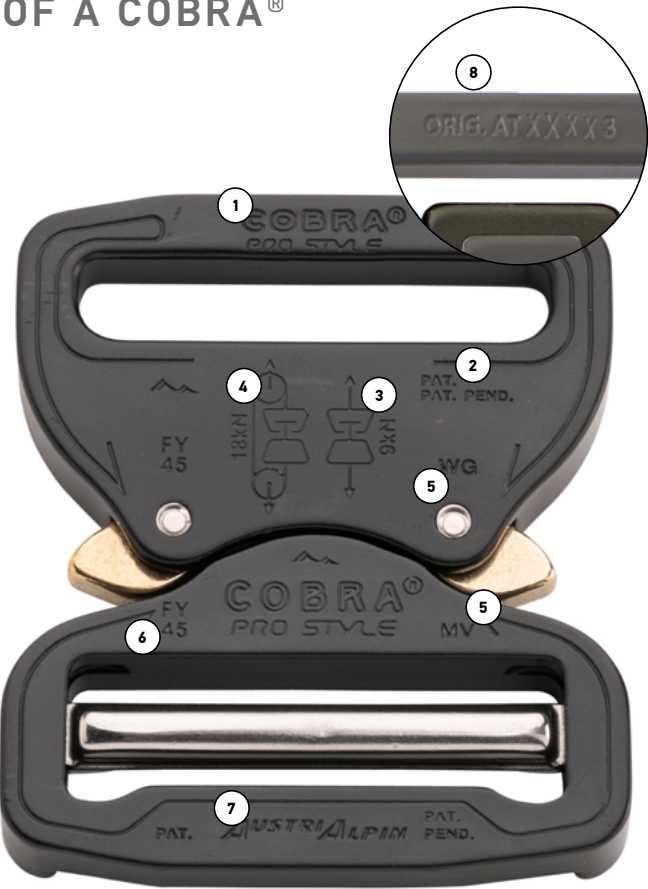
VORDERSEITE FRONT
